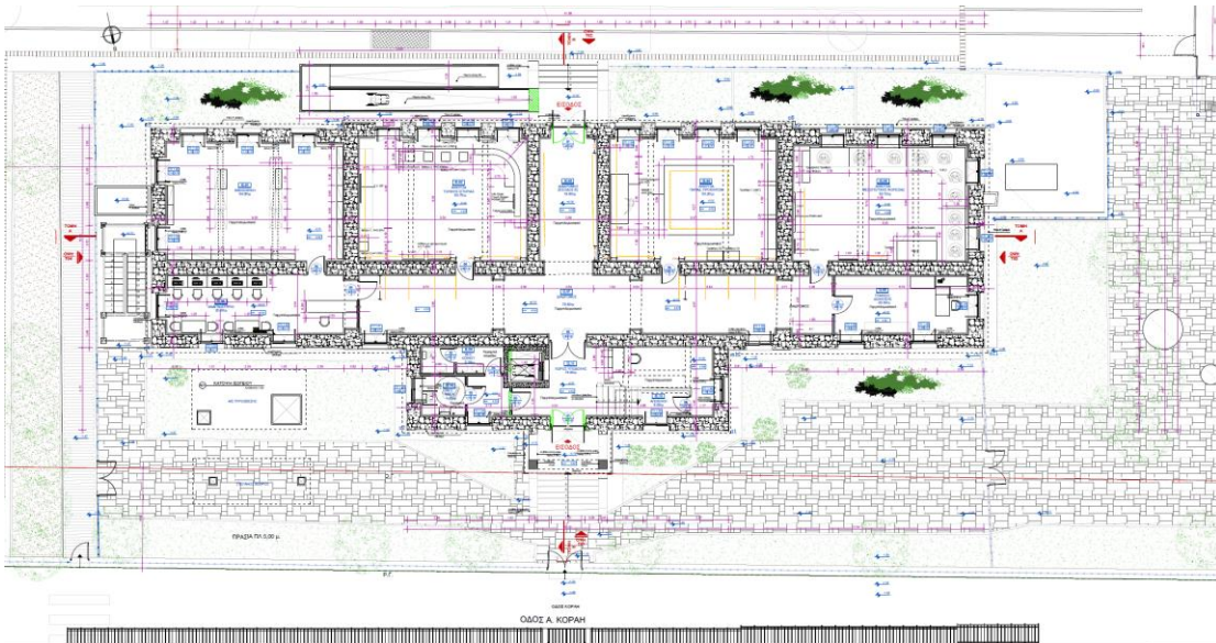
Εικόνα 9: Κάτοψη ισογείου – αίθουσα Μεσογείτικης φορεσιάς
